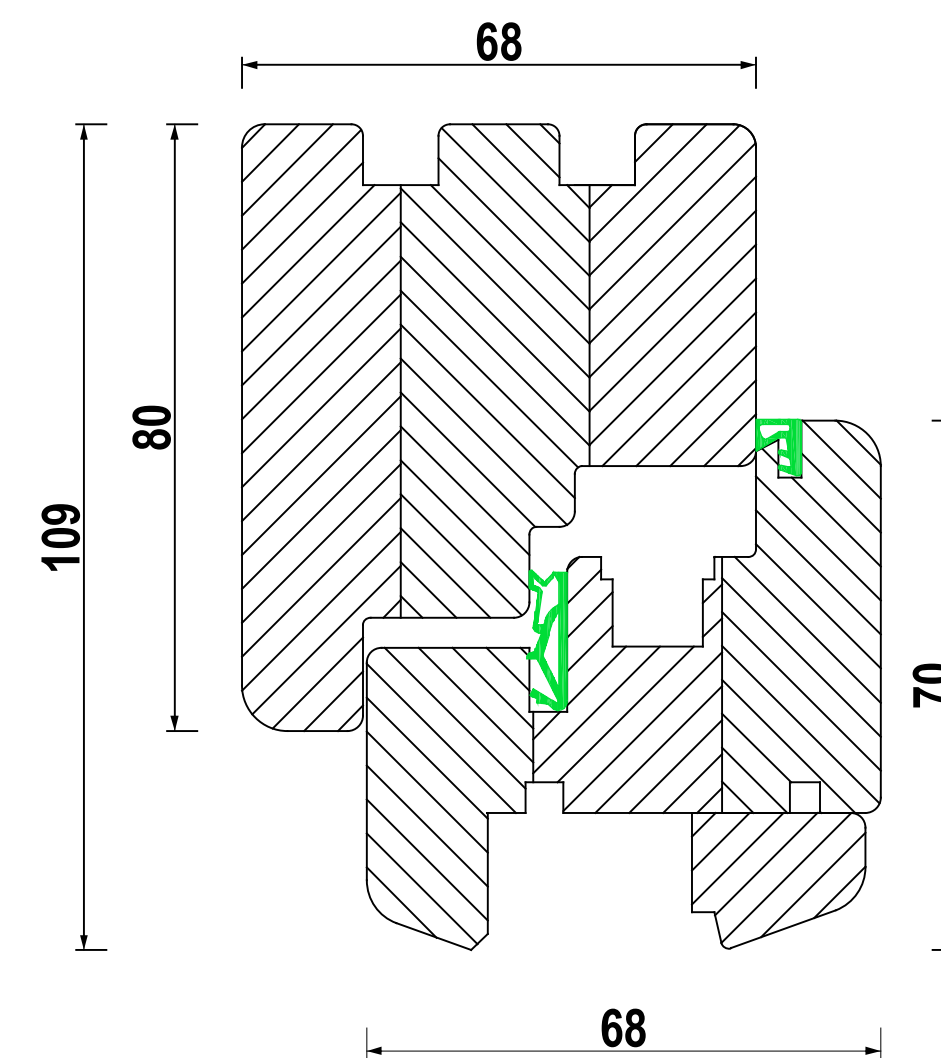
RAHMEN O+L+R 80mm FLÜGEL 70mm
