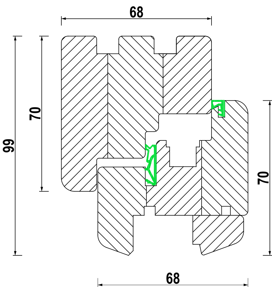
RAHMEN O+L+R 70mm FLÜGEL 70mm
