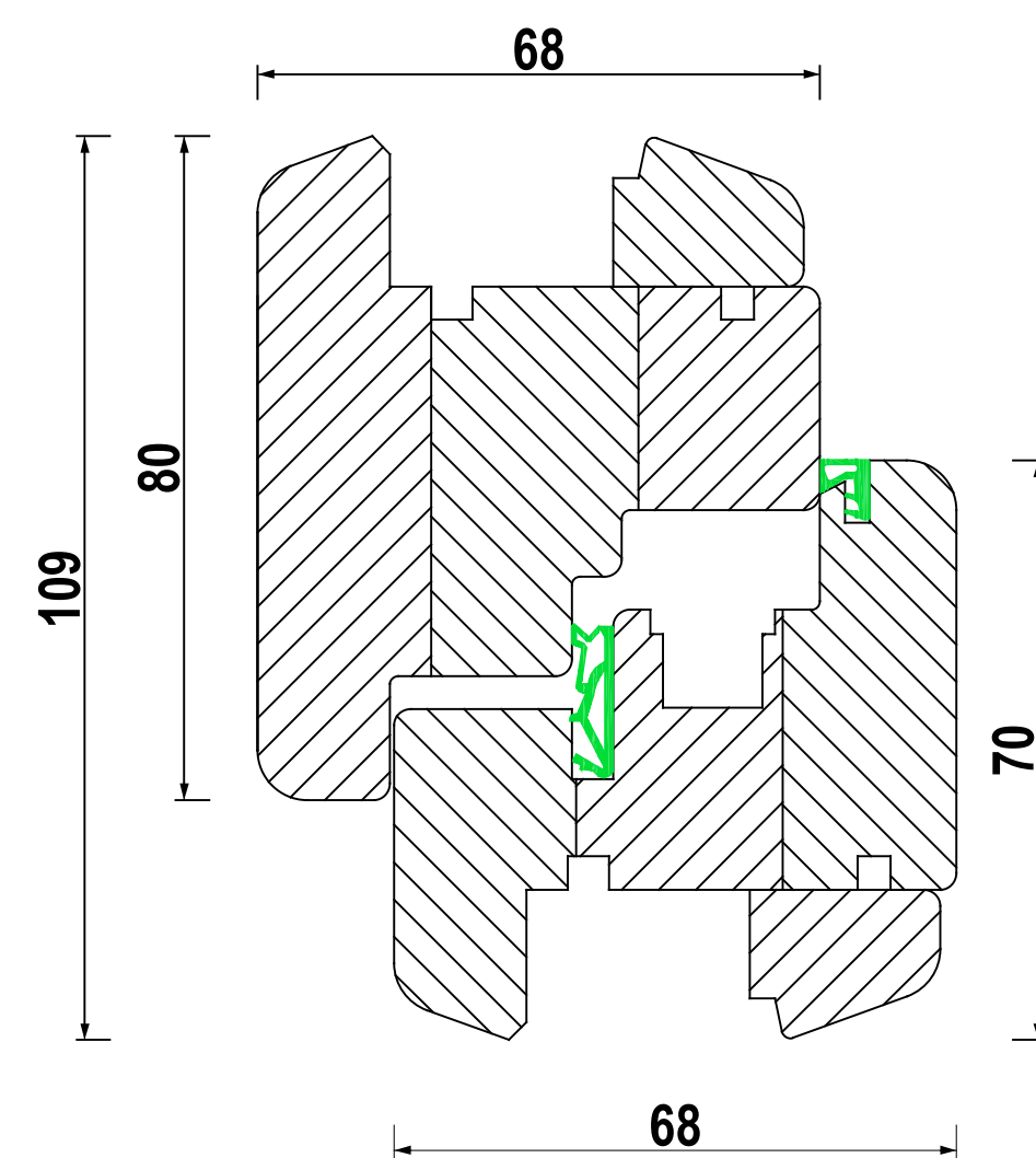
FIX OBEN 80mm FLÜGEL 70mm
