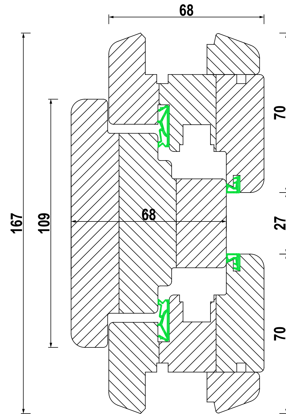
PFOSTEN 109mm FLÜGEL 70mm
