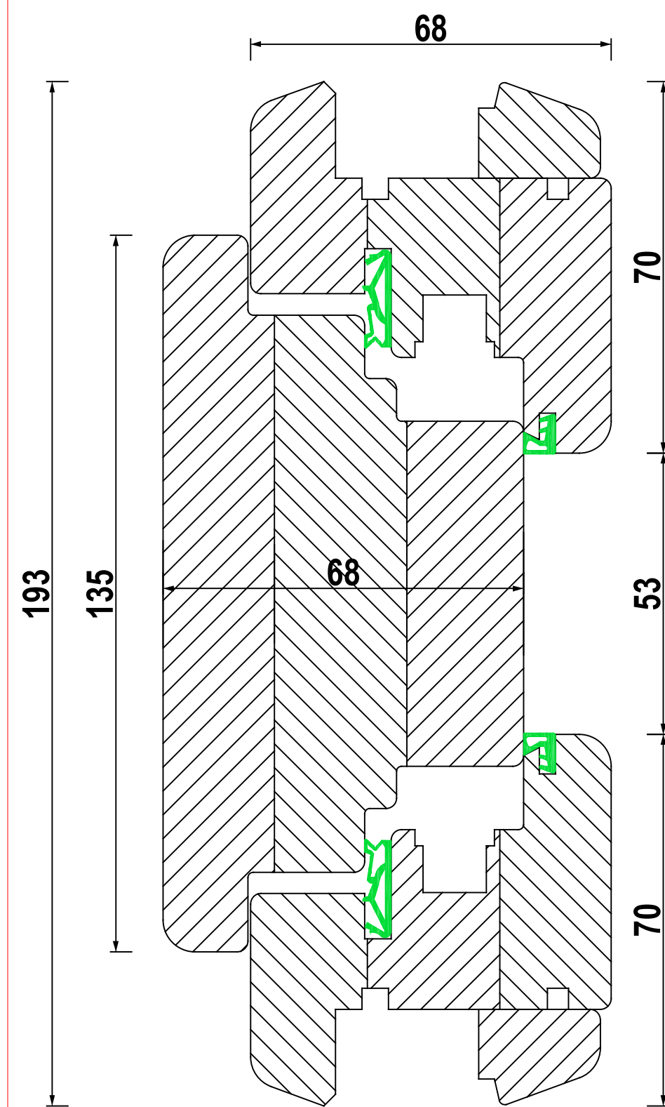
PFOSTEN 135mm FLÜGEL 70mm
