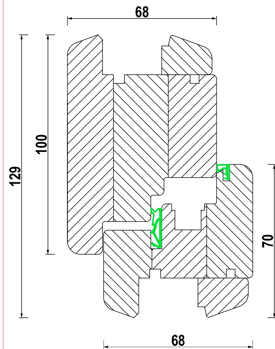
FIX OBEN 100mm FLÜGEL 70mm
