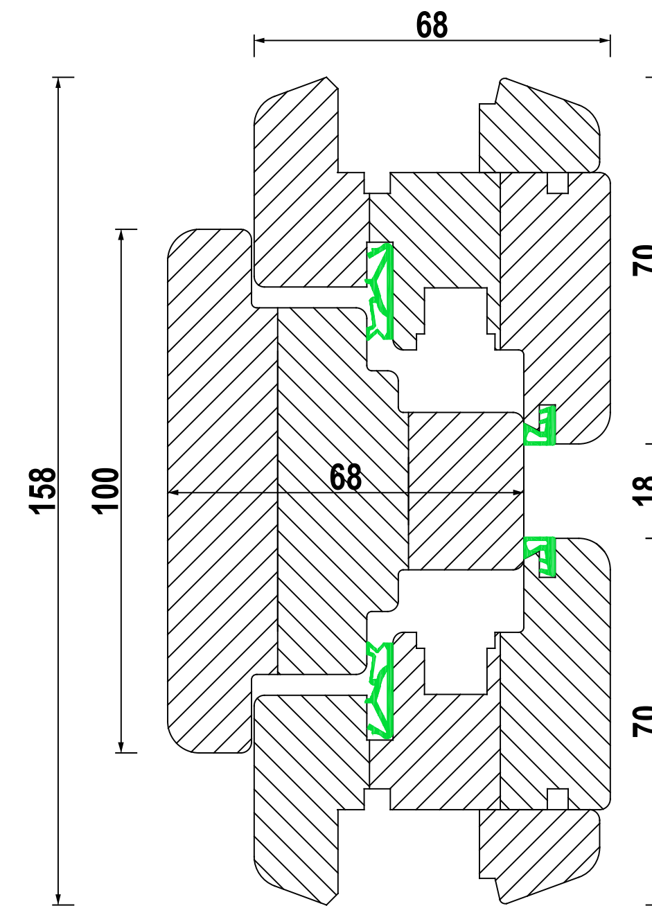
PFOSTEN 100mm FLÜGEL 70mm
