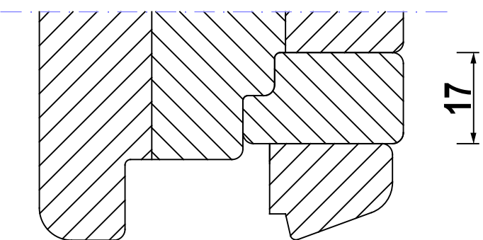
FIX ELEMENT (O+L+R) AUSGLEICH
