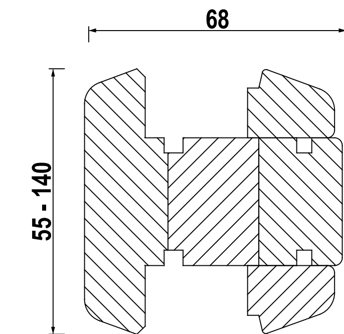
GLASTEILENDE SPROSSE
